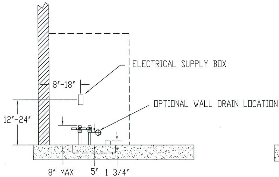
VIEW A-A
